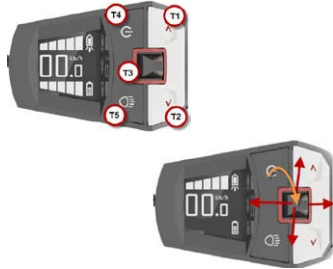
Abb. 2 Tasten und Joystick der Bedieneinheit Comfort
